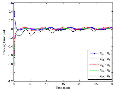
5(a). Tracking error
